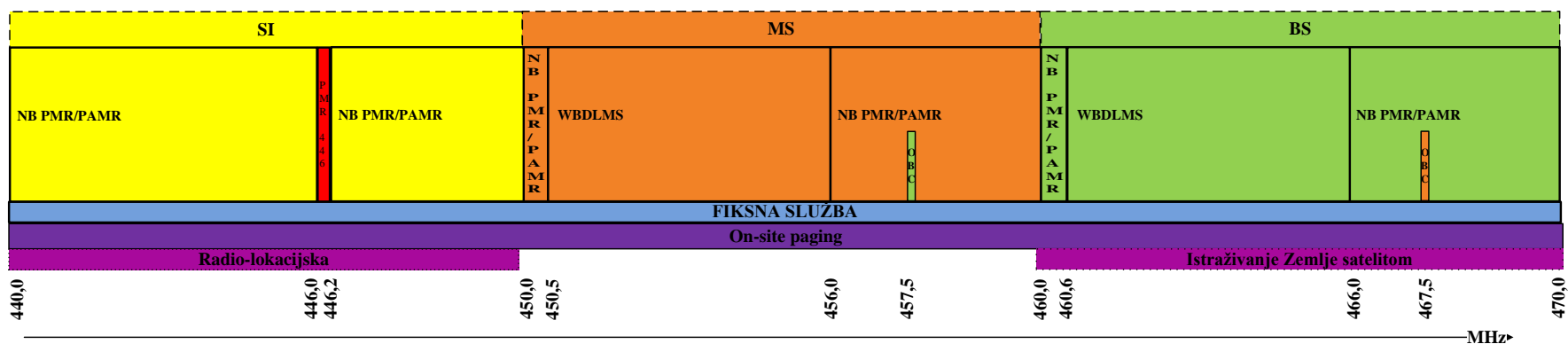
Slika 1: Grafički prikaz raspodjele opsega 440-470 MHz
